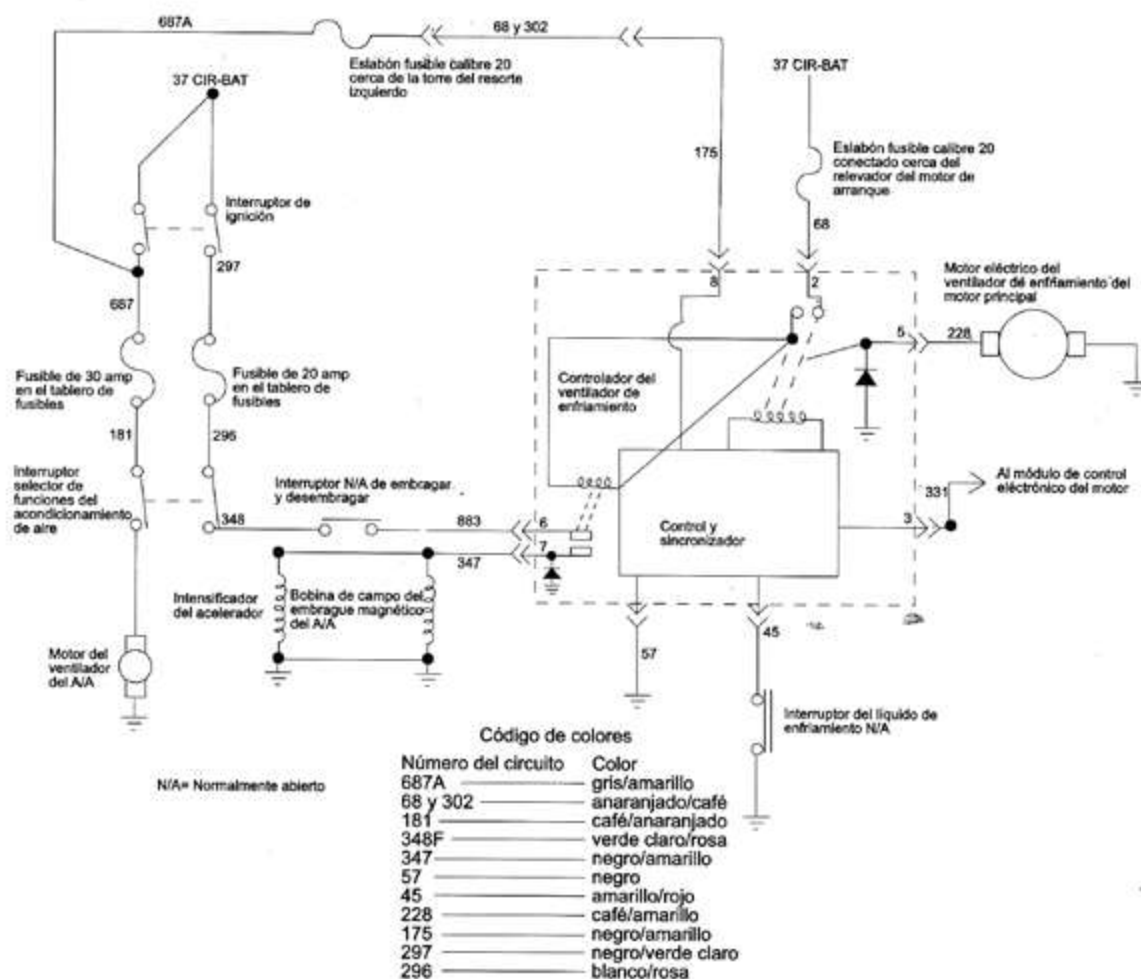
Diagrama de flujo de corriente
